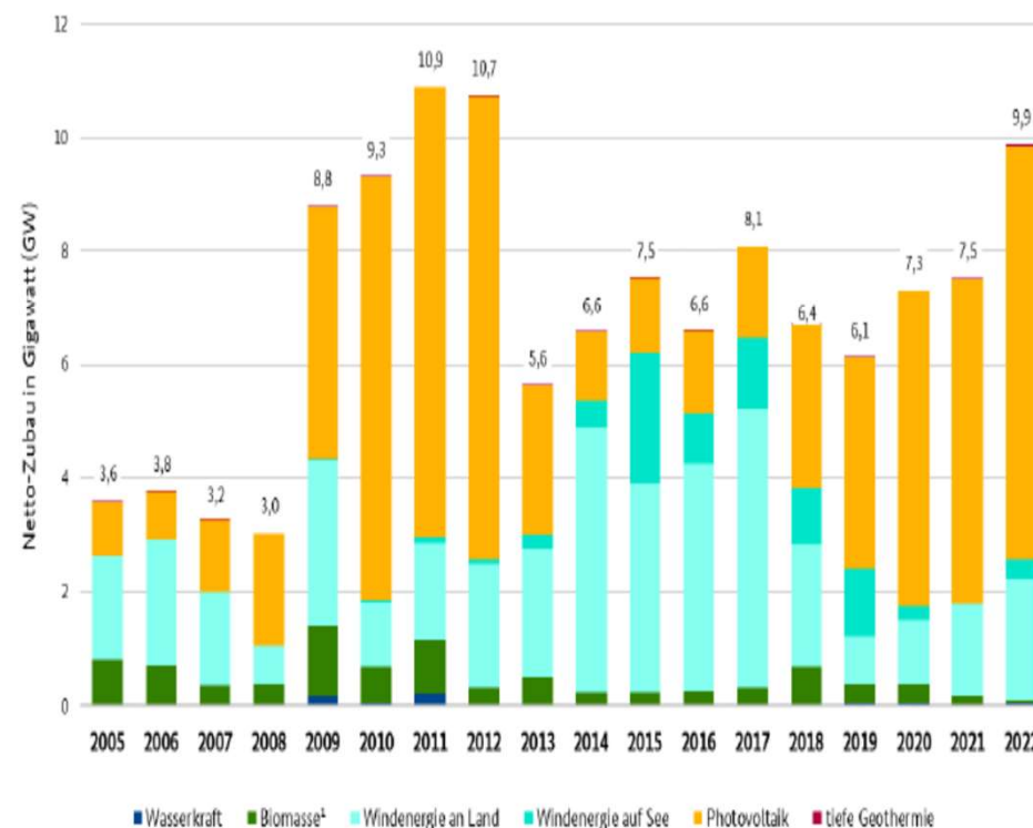
Entwicklung des Netto-Zubaus an installierter Leistung zur Stromerzeugung aus Erneuerbaren Energien in Deutschland
